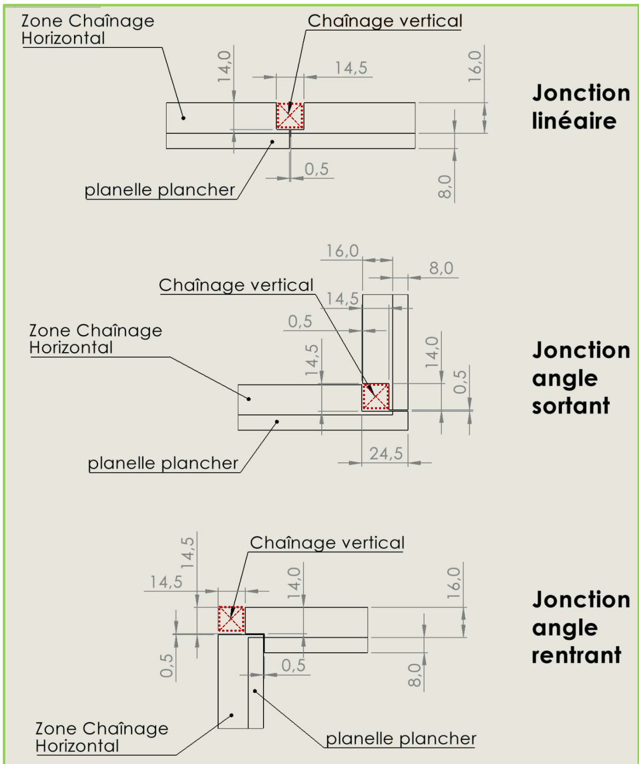
Figure 11 Détails jonctions de panneaux 24cm
