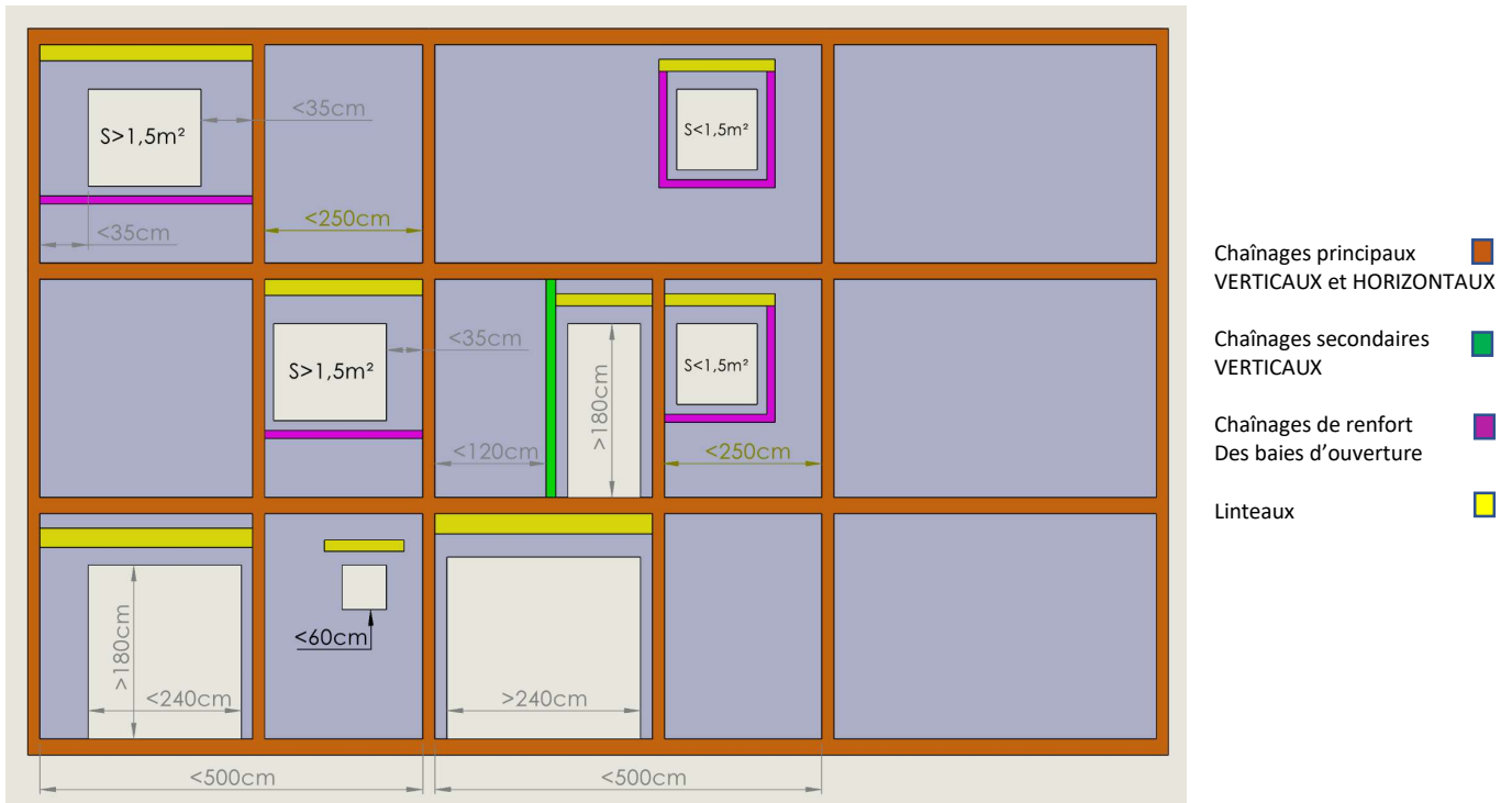
Figure A29 : Dispositions de principe des chaînages pour les configurations D, E et F – hors analyse de structure ou exigences particulières :
