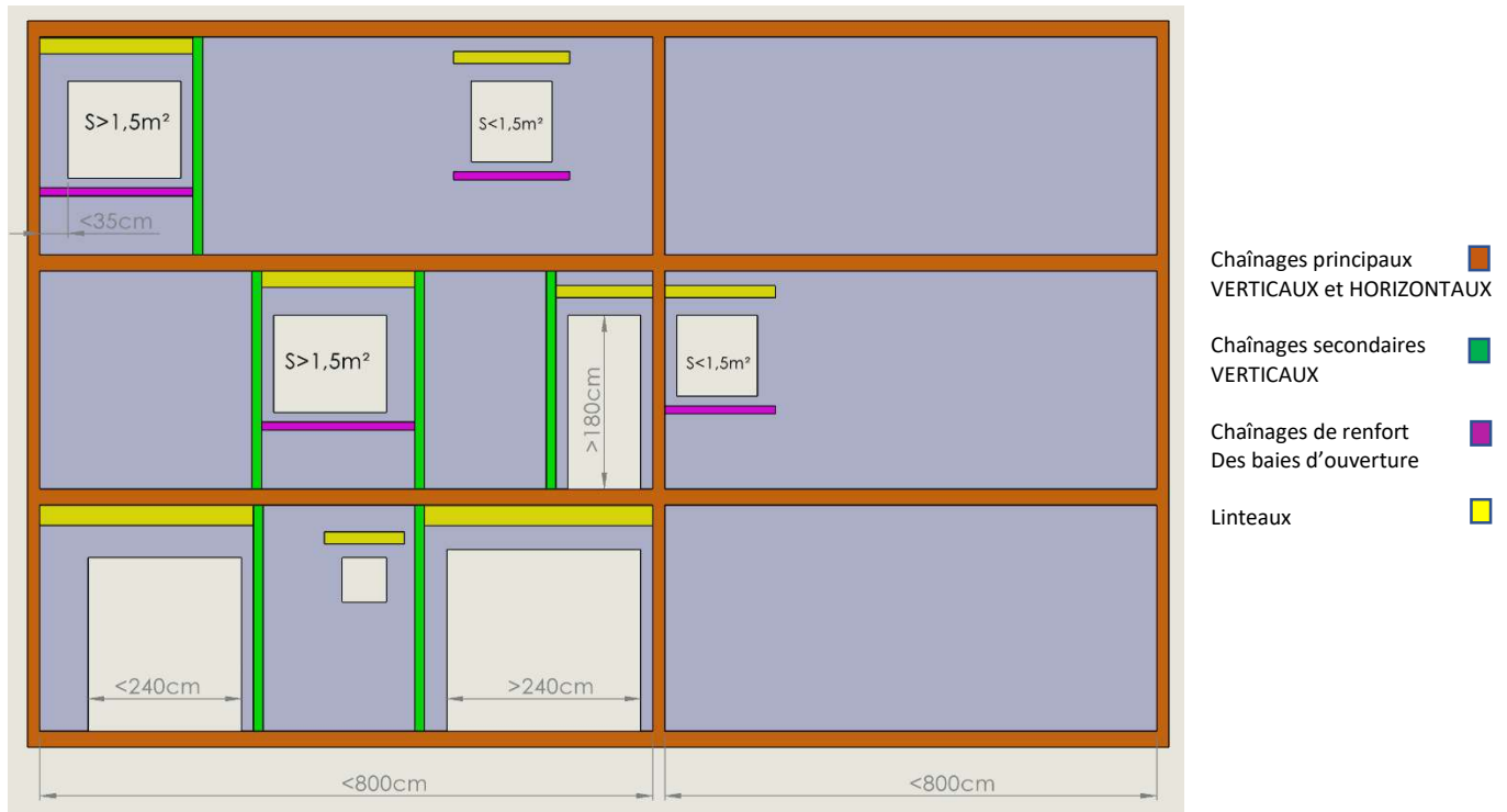
Figure A27 : Dispositions de principe des chaînages pour la configuration A, zones sismiques 1 et 2 – hors analyse de structure :
