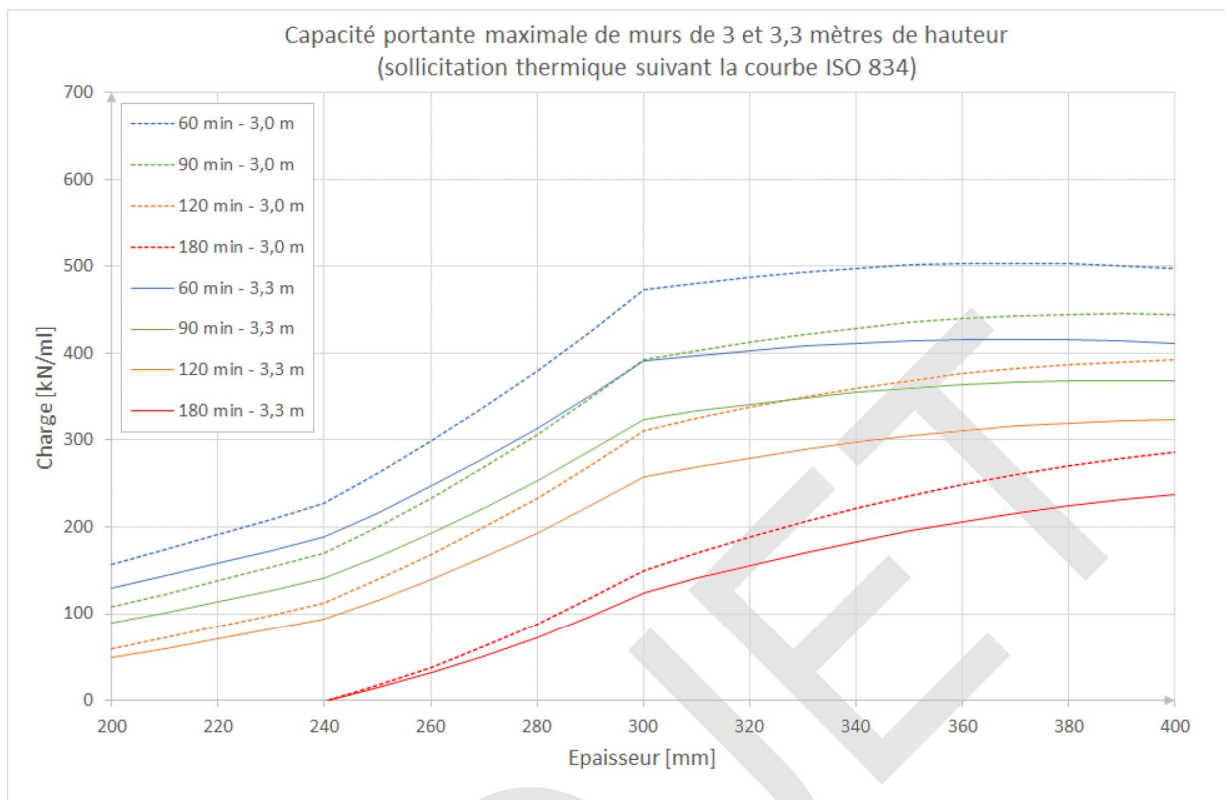
Figure 5.2 : Capacité portante des murs porteurs considérés selon l'épaisseur et la performance au feu recherchée
