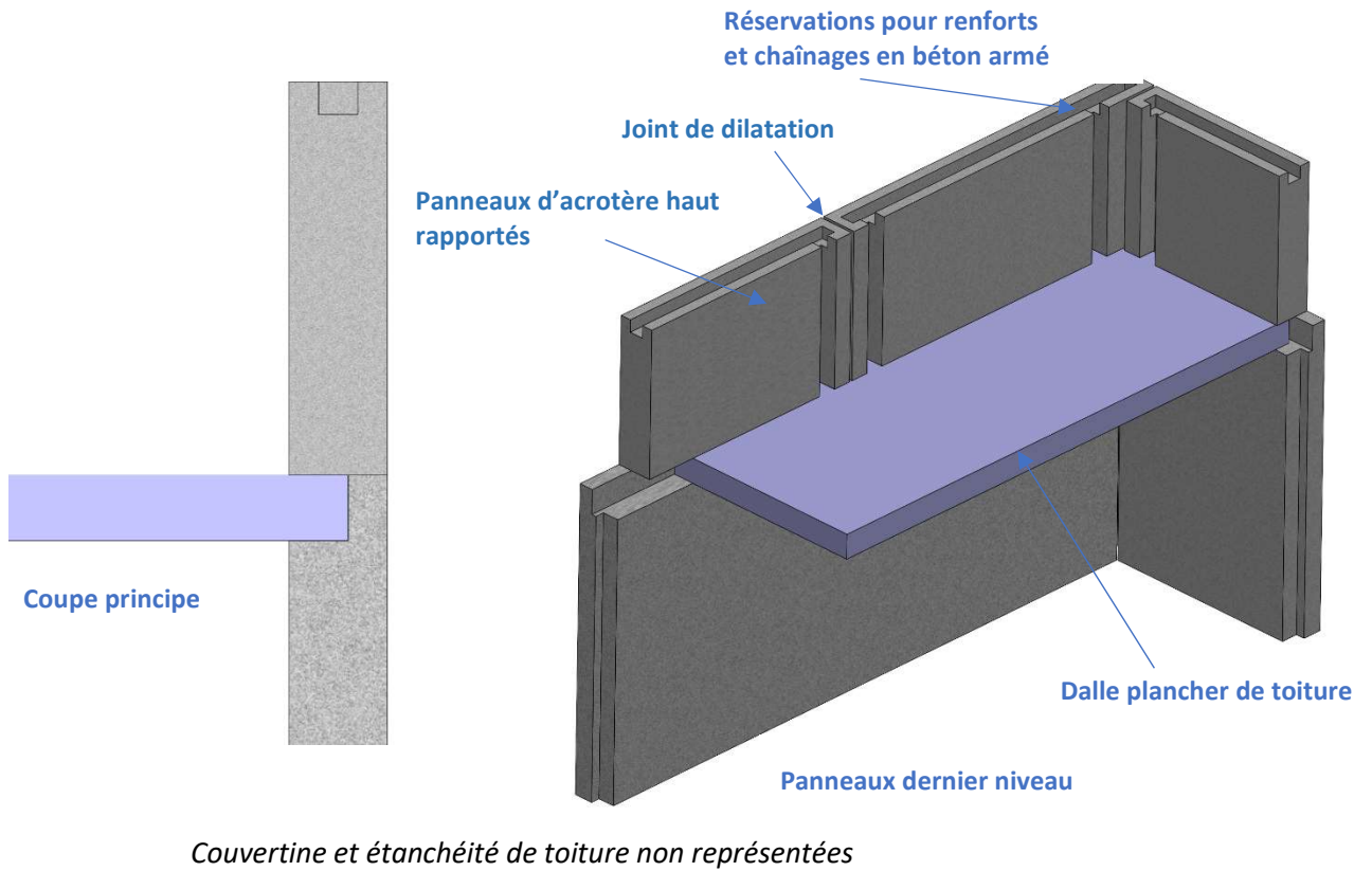
Figure A25-C : Acrotère haut rapporté sur dalle toiture
